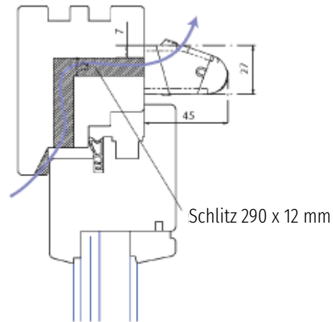
Abb. 16: Feuchtegeführter Luftdurchlass für Holzfenster (Maße bzw. Fräsung typbeding) Quelle: Aereco GmbH
