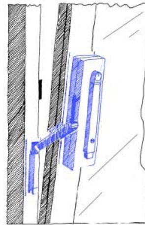
Abb. 15: Fensterkippmotor
