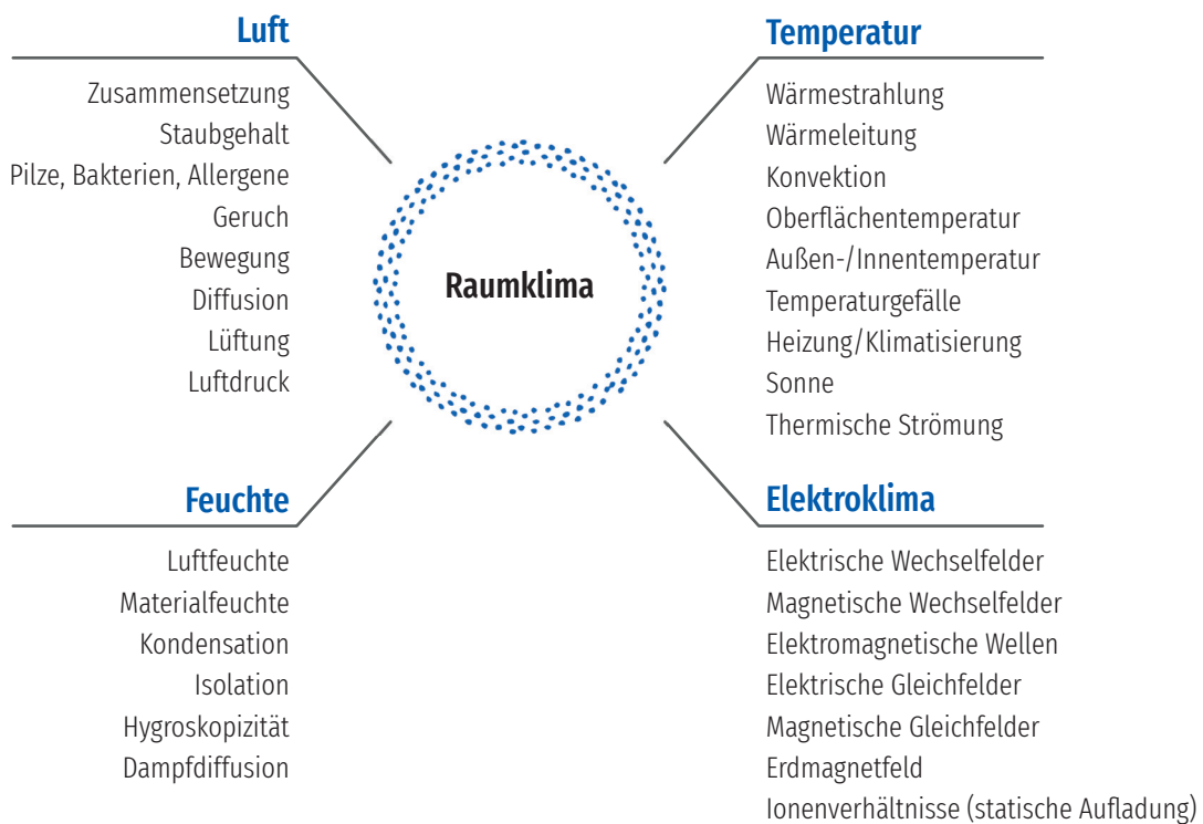
Abb. 02: Klimafaktoren in Häusern
