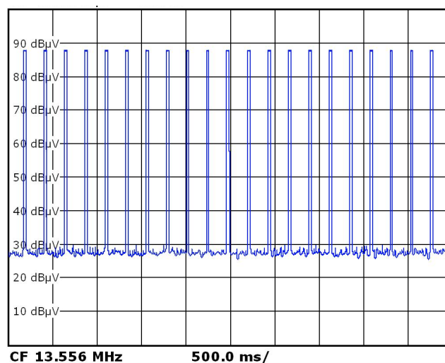
Abb. 7: NFC-Puls der Toniebox auf der Frequenz 13,56 MHz; Aufzeichnung mit einem konventionellen Spektrumanalysator in der Betriebsart „Zero Span“ (Zeitdarstellung), Zeitachse 500 ms/Teilung = 5 s
