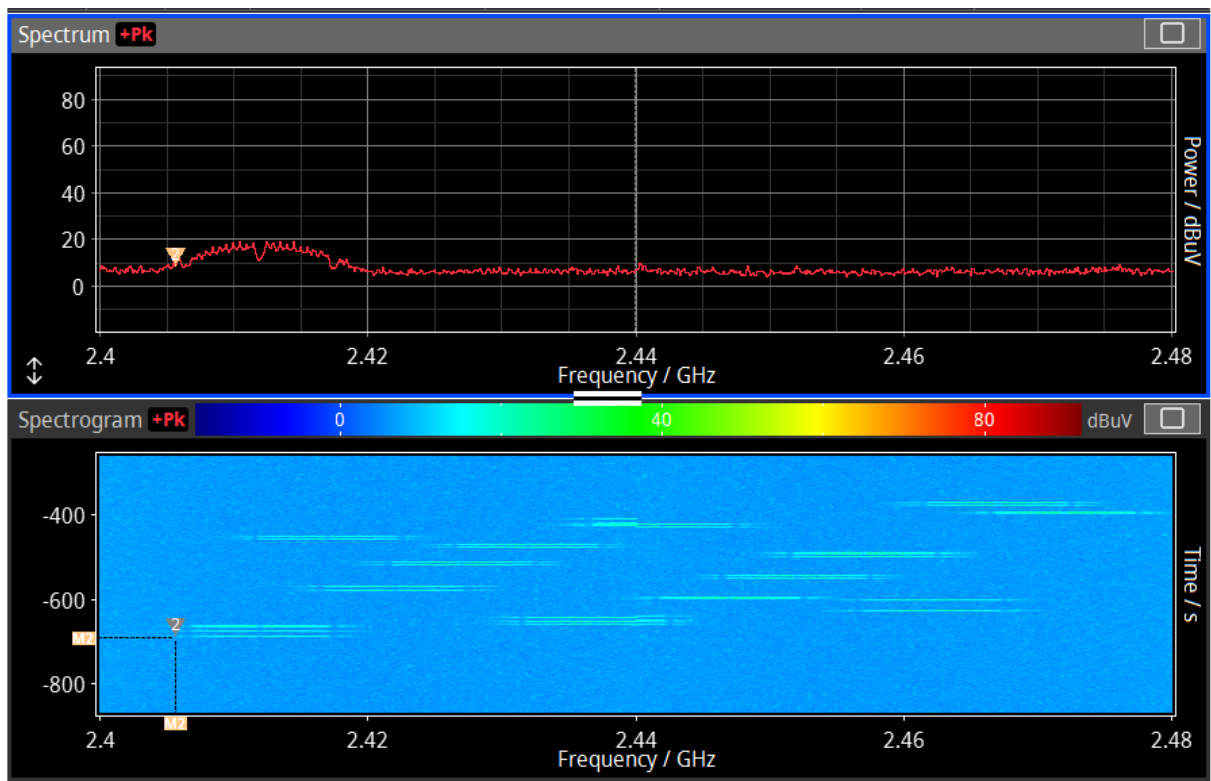
Abb. 5b: WLAN-Burst, mit größerer zeitlicher Auflösung im Spektrogramm (unten, Zeitachse 600 ms = 0,6 s) und Anzeige im Spektrum (oben) ohne Maximalwert-Speicher. Im Spektrogramm sind nun die zeitliche Abfolge der Impulse und die Verteilung über das WLAN-Band noch deutlicher zu erkennen; die Dauer des Bursts beträgt ca. 300 ms. Im Spektrum wird jetzt nur der Anteil eines einzelnen Bursts, und zwar an der Stelle des Markers (gestrichelte Linien M2) dargestellt. Die Signalbandbreite beträgt ca. 16 MHz.
