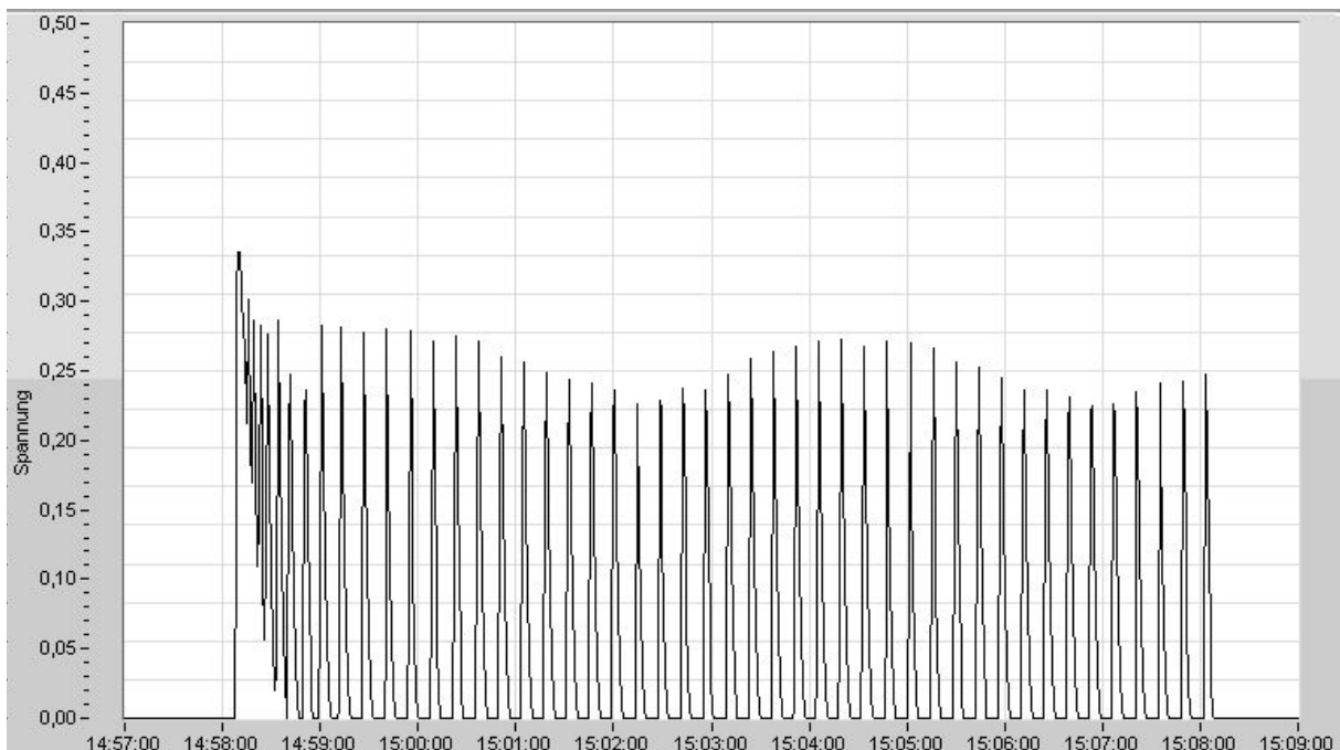
Abb. 4: Aussendung der WLAN-Bursts über 10 Minuten; Aufzeichnung der Ausgangsspannung eines HF-Breitbandmessgerätes mittels Datenlogger
