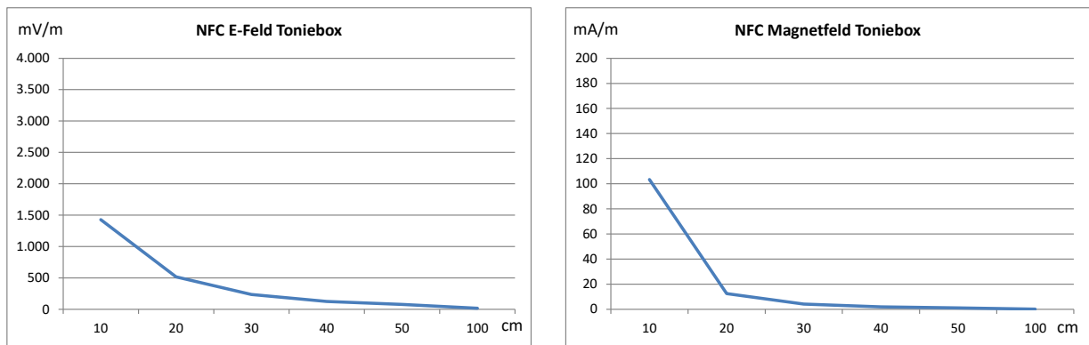
Abb. 8: Elektrische (links) und magnetische (rechts) Feldstärke des NFC-Signals als Funktion des Abstandes von der Toniebox (gemessen mit Spektrumanalysator und Peak-Detector, Spitzenwert)
