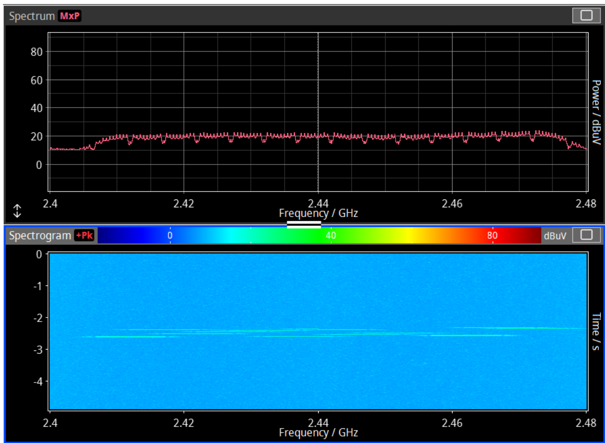
Abb. 5a: WLAN-Burst, dargestellt mit einem Realtime-Spektrogramm (oben) und als so genanntes Spektrogramm (unten).
